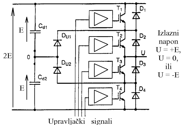
Slika 3.3.3: Jedna faza višenivskog invertora za napajanje motora za naizmeničnu struju srednjeg naponskog nivoa.
