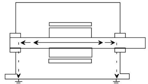
Slika 3.3.2: Uspostavljanje parazitarne kružne struje kroz kućište i ležajeve motora napajanog iz frekvencijskog regulatora.
