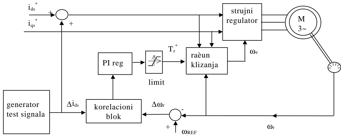
Slika 2.6.2.1: Identifikacija električnih parametara rotorskog kola asinhronog motora zasnovana na injektovanju test signala u struju magnetizacije.
