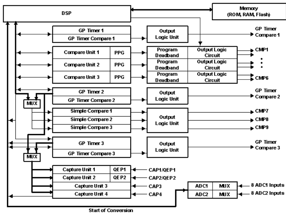
Slika 2.8.2: Primer objedinjavanja digitalnog procesora i A/D konvertora u jedinstvenom integrisanom kolu (320F240 [22]).
