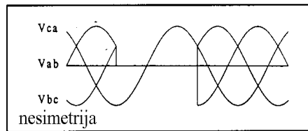
Slika 3.3.1: Vrste kratkotrajnih neregularnosti mrežnog napona pri kojima se još uvek očekuje ispravan rad pogona.
