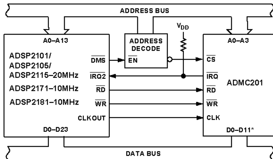
Slika 2.8.3: Primer realizacije pogonskog kontrolera sa razdvajanjem analognih i digitalnih funkcija u dva kola [149].
