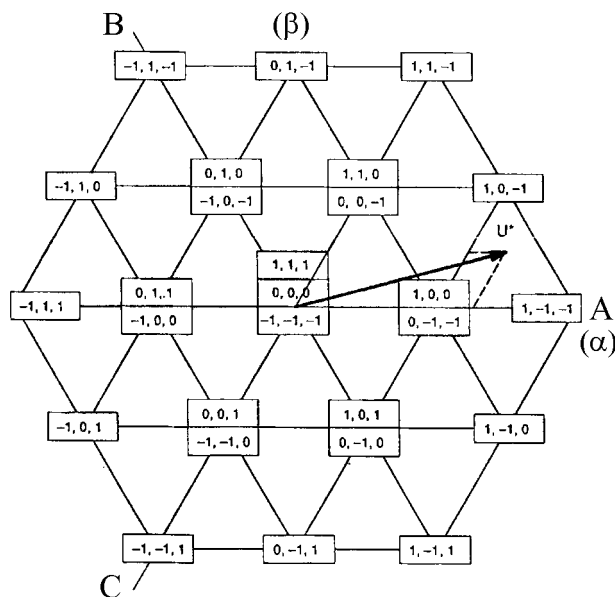
Slika 3.3.4: Raspoloživi vektori izlaznog napona trofaznog višenivskog pretvarača za motore srednjih napona. U svakoj fazi postoje tri diskretne vrednosti (-E, 0, +E) pa je broj vektora 19 (konvencionalni inverter može dati 7 različitih naponskih vektora).
