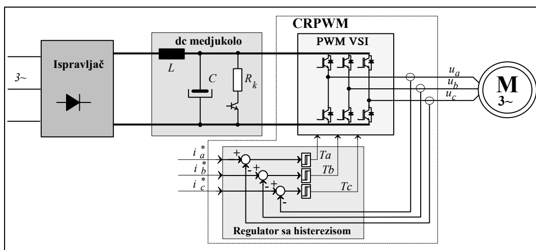
Slika 2.6.4.2: CRPWM Current Regulated Pulse Width Modulated VSI Trofazni inverter sa lokalnom povratnom spregom po struji i analognim strujnim regulatorom koji primenjuje komparatore sa histerezisom.
