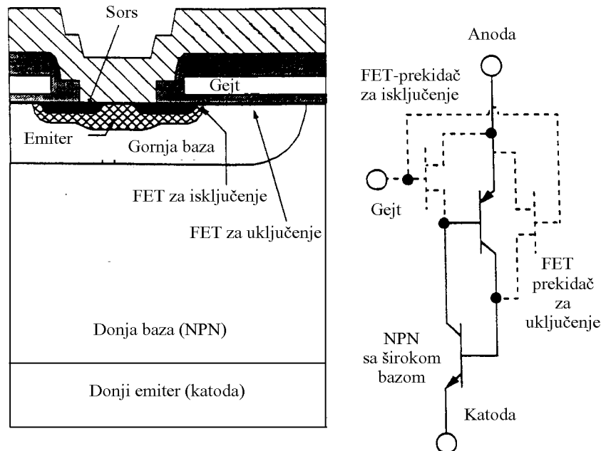
Slika 3.4.1: Način izrade i ekvivalentna šema MCT prekidača.
