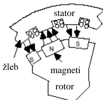
Slika 2.6.3.3: Valovitost momenta usled interakcije magneta i statorskih žlebova ( cogging detent torque ).
