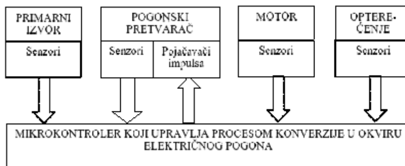
Slika 2.8.1: Funkcije digitalnog pogonskog kontrolera.
