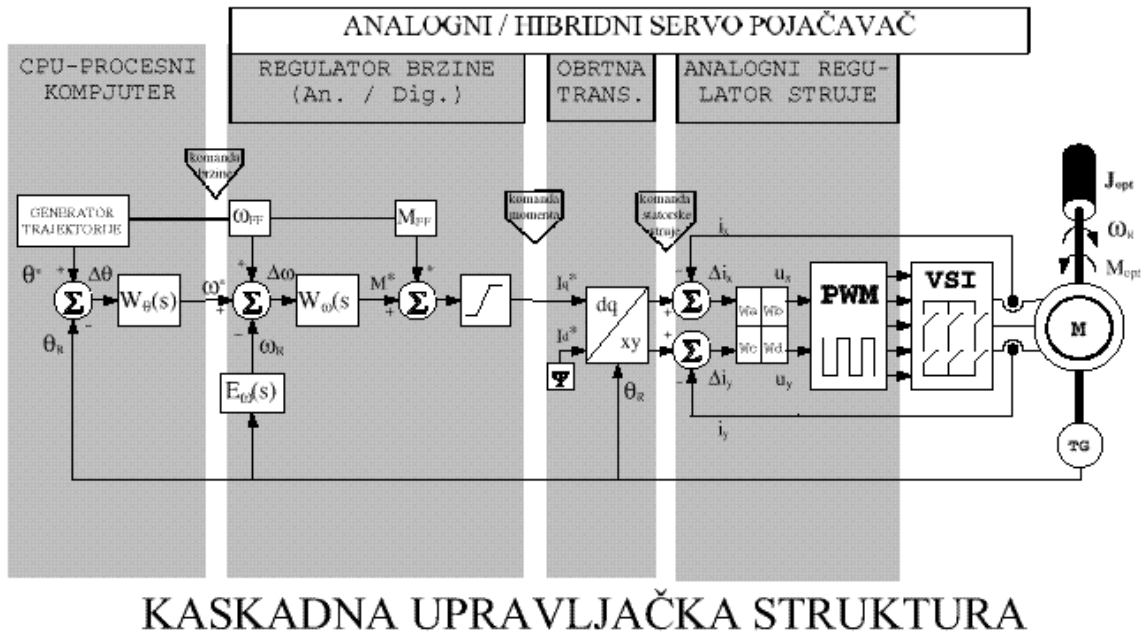
Slika 2.5.2. Kaskadna struktura pogonskog kontrolera kod servopojlašavačkog modula namenjenog korišćenju u centralizovanom sistemu za kontrolu kretanja. Regulator položaja je fizički razdvojen (CNC) od regulatora struje i brzine (servopojlašavač).
