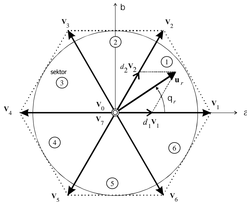
Slika 2.6.4.4: DTC momentni modulator za svaki komutacioni interval vrši selekciju sekvence naponskih vektora tako da se minimizira kriterijumska funkcija najčešće kvadratno odstupanje fluksa i momenta od željenih vrednosti. Sekvenca ilustrovana na slici uključuje vektore V_1 (100), V_2 (110) i V_0 (000).
