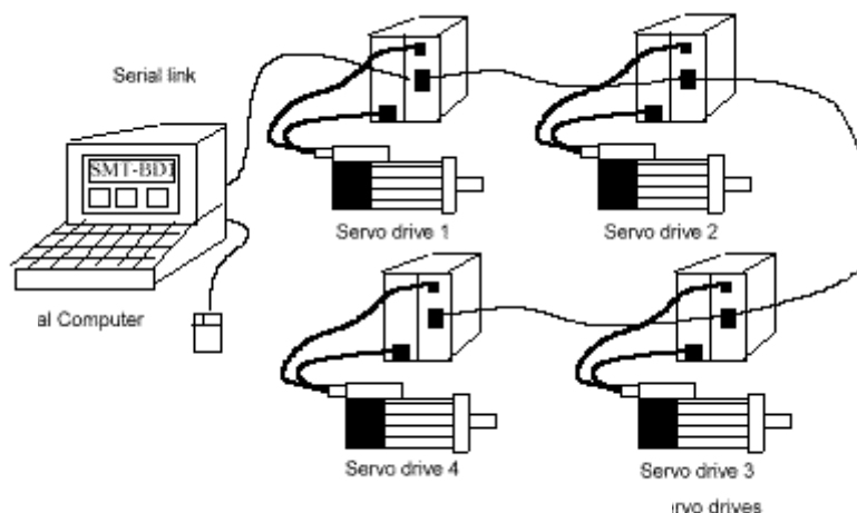
Slika 2.7.2: Četveroosni servo sistem sa digitalnom komunikacijom između računara i servo pojačavača: jedinstvene sabirnice umanjuju broj veza.
