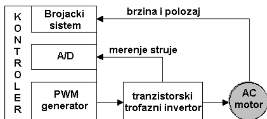
Slika 1.1: Osnovne funkcije merenja i upravljanja digitalnog kontrolera u pogonu sa asinhronim motorom.
