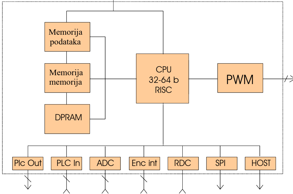
Slika 2.7.5: Servoprocetor podesan za izvršavanje Motion Control Basic programa.
